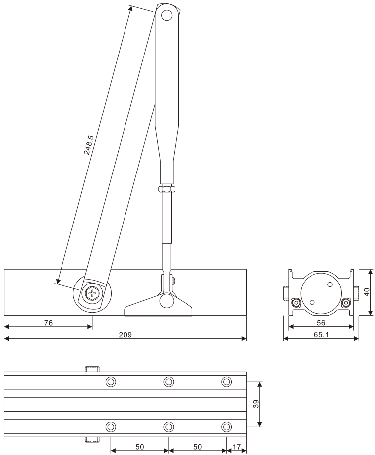
外形尺寸/Overall dimension
