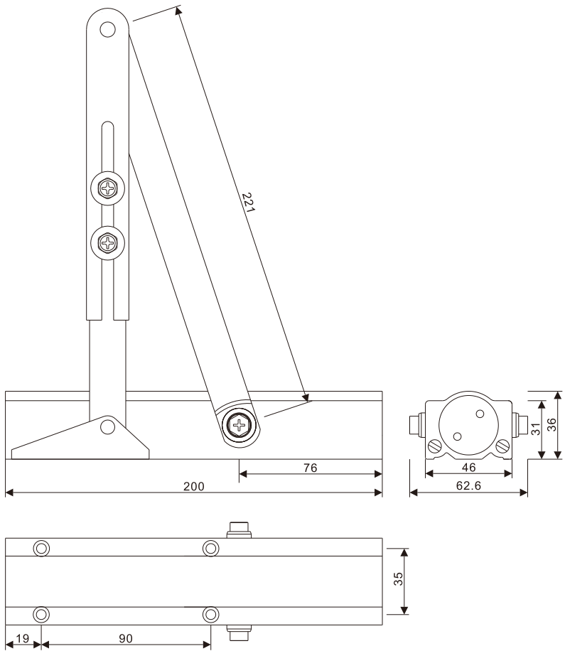
外形尺寸/Overall dimension
