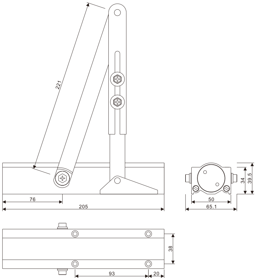
外形尺寸/Overall dimension
